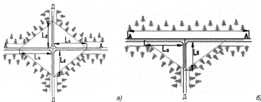
а) - на пересечениях автомобильных дорог в одном уровне; б) - на примыканиях автомобильных дорог в одном уровне
