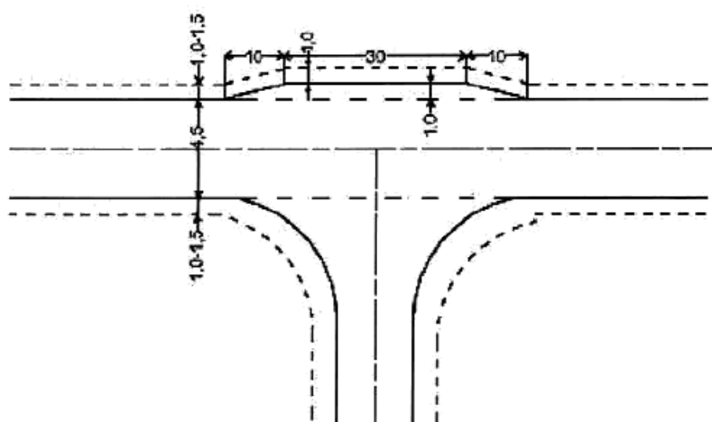
в) Карман в зоне примыкания
